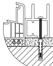
DETAIL UCHYCENÍ VODÍCÍ LIŠTY
