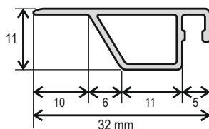
Příčka
