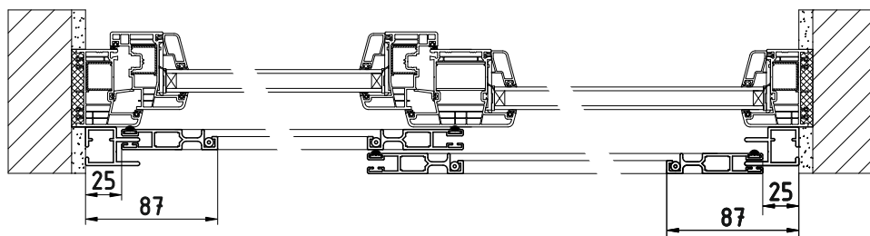
PŮDORYS:
