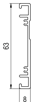
PŘÍČKA
