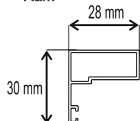
Profil pro kartáček
