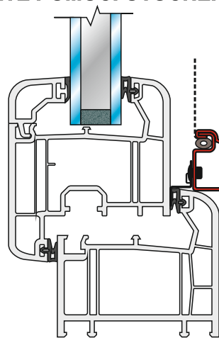
VNĚJŠÍ ROH
