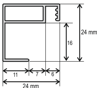
Příčka
