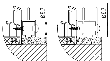
DETAIL UCHYCENÍ VODÍCÍ LIŠTY
